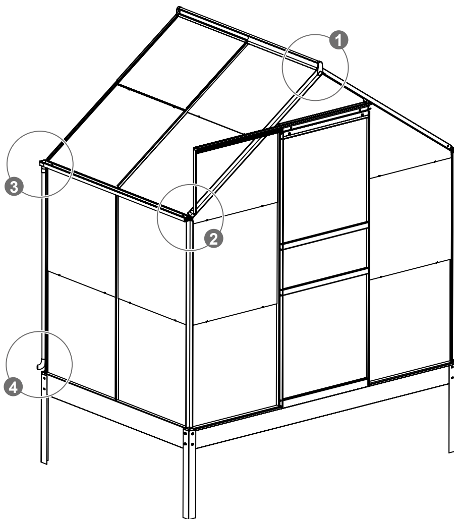
Détail embout de faîtière (pièce 2010) Abdeckung der Firstspitze (Einzelteil 2010) Roof ridge end cover (part 2010)
