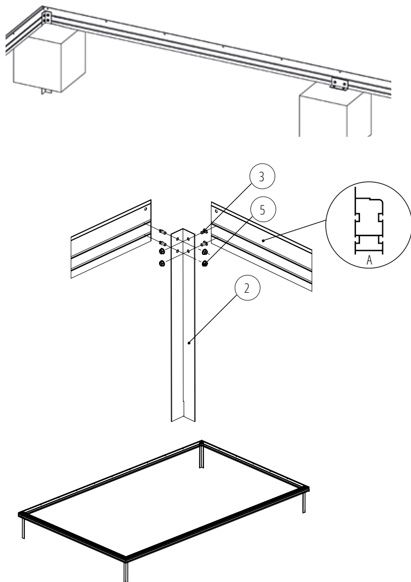
Montage final
